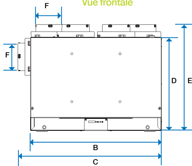
Vue frontale
