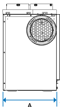
Vue latérale
