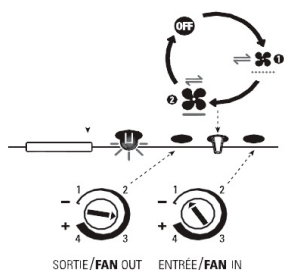
Détail des potentiomètres sur le VRE
