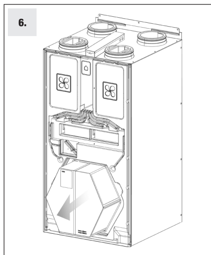
Retirer le noyau de récupération en tirant lentement.
