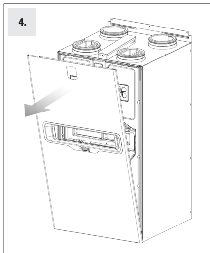
Faire basculer la porte vers l'avant et la soulever.
