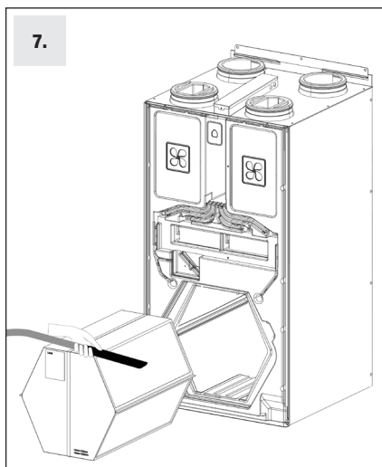
Nettoyer le noyau de récupération avec un aspirateur (pas d'eau ni de solvants).
