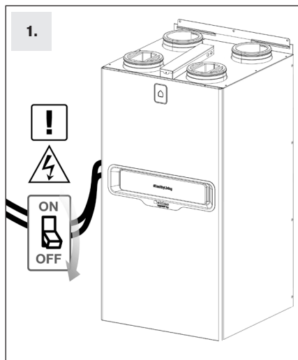
Couper le courant.
