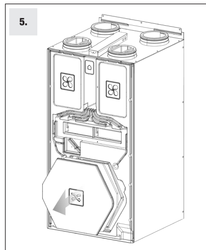
Enlever le couvert du noyau de récupération.
