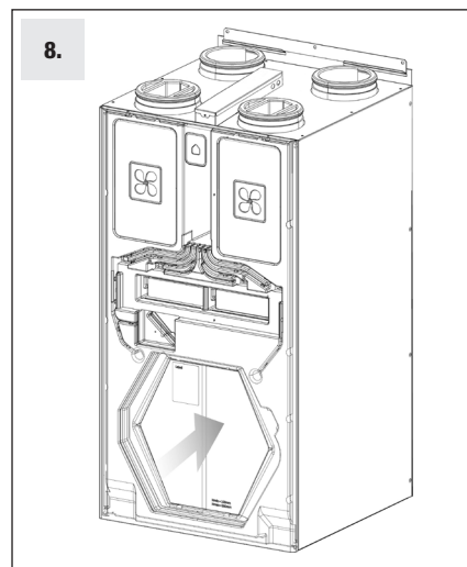
Remettre en place le noyau de récupération en le poussant horizontalement avec précaution.
