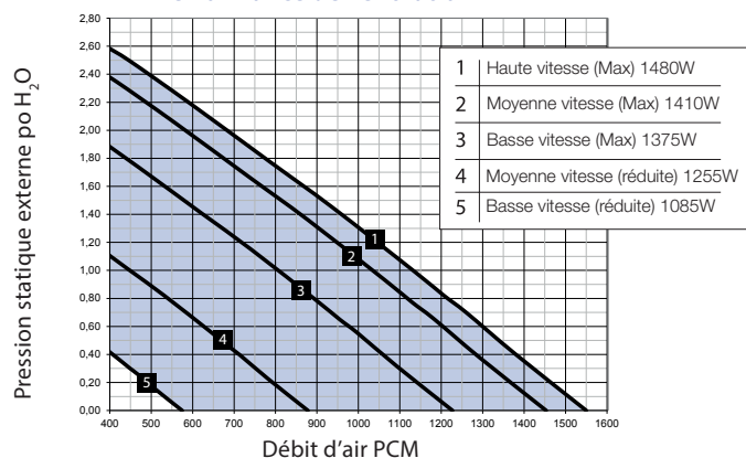
E1800L-Fi-N Performance de ventilation
