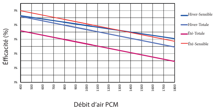
E1800L-Fi-N Efficacité du noyau
