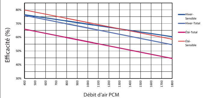
E1800L-Fi-EC-N Efficacité du noyau
