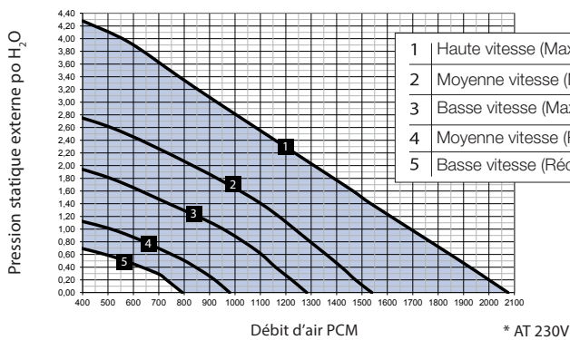
E1800L-Fi-EC-N Performance de ventilation
