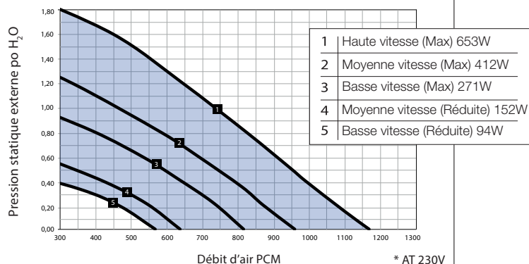
E1100L-Fi-EC-N Performance de ventilation
