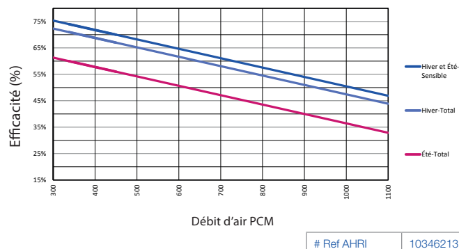
E1100L-Fi-EC-N Efficacité du noyau
