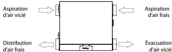
VERSION INVERSEE E130-HR-M
