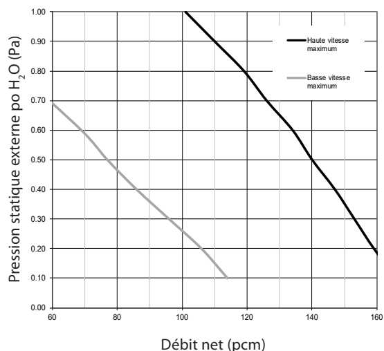
E130-HRX Performance de Ventilation
