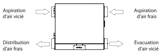
VERSION INVERSEE E130-HRX-M
