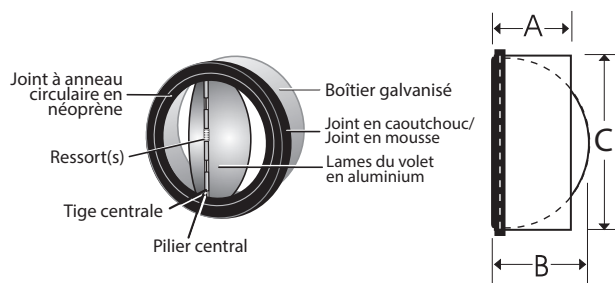
MODÈLES 4" - 7" MANCHON EN MÉTAL ESTAMPÉ/DESIGN DE LA TIGE CENTRALE
