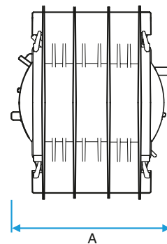
VUE LATÉRALE
