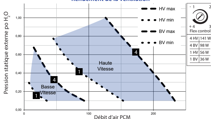
H190-TRG Rendement de la ventilation
