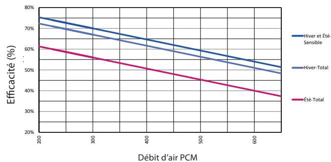
E650L-Fi-EC-N Efficacité du noyau
