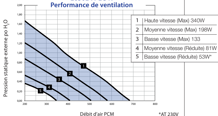
E650L-Fi-EC-N Performance de ventilation
