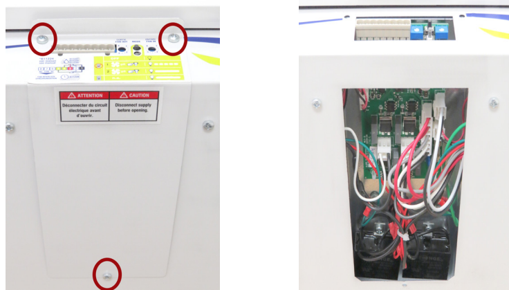
Enlèvement des vis
