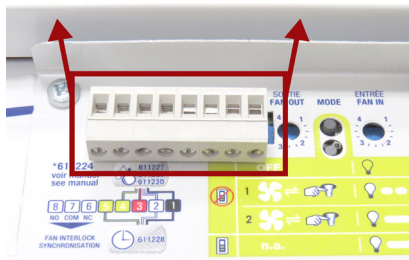
Enlèvement du bornier de l'appareil
