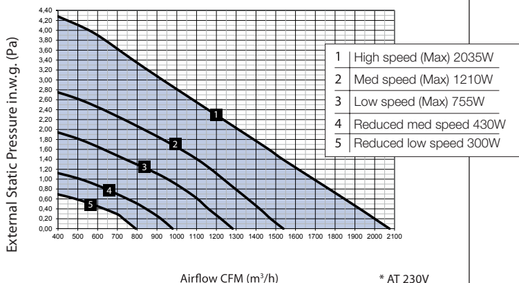
E1800L-Fi-EC & E1800L-Ri-EC Ventilation Performance
