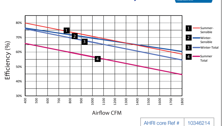
E1800L-Fi-EC & E1800L-Ri-EC Core Efficiency
