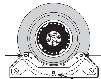
Montage du support et localisation des vis
