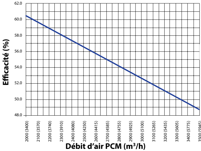
CH3000 - Efficacité sensible du cube en polypropylène
