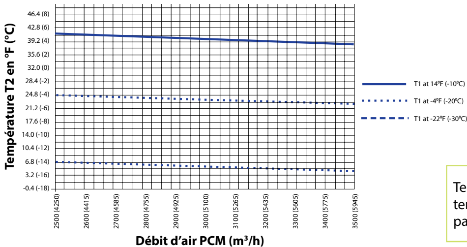
Température d'alimentation T2 (T3 à 70°F BS / 58°F BH) avec volet de face et d'évitement
